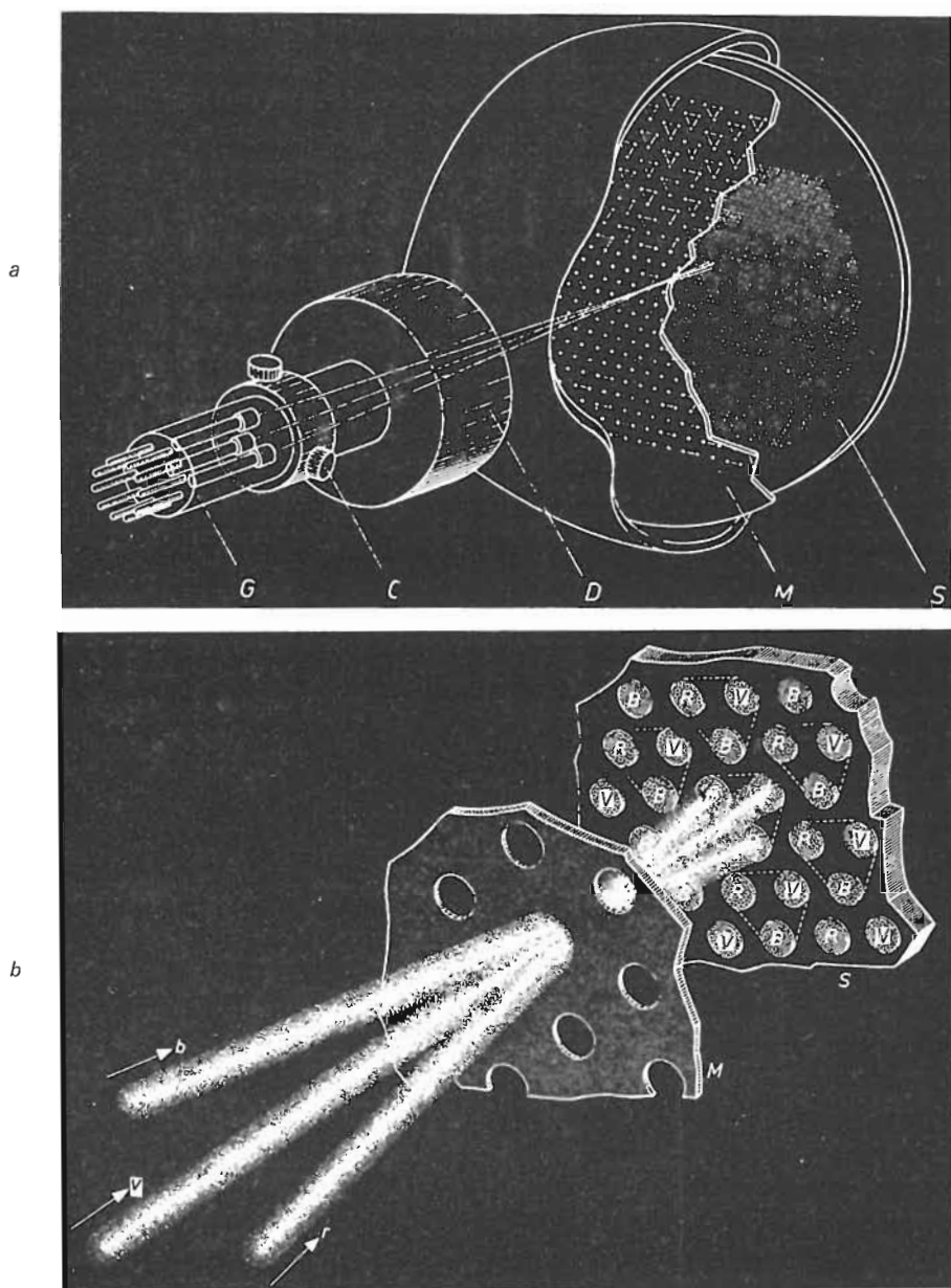
Figura 27. - Cinescopio a maschera. - a) sezione; b) dettaglio ingrandito dei tre pennelli elettronici che passano attraverso la maschera; b , v , r = pennelli elettronici per i puntini luminosi blu, verde e rosso; C = sistema di convergenza; D = sistema di deflessione; G = base del tubo con i tre cannoni elettronici; M = maschera; S = schermo luminescente sotto forma di terne di punti luminosi.
